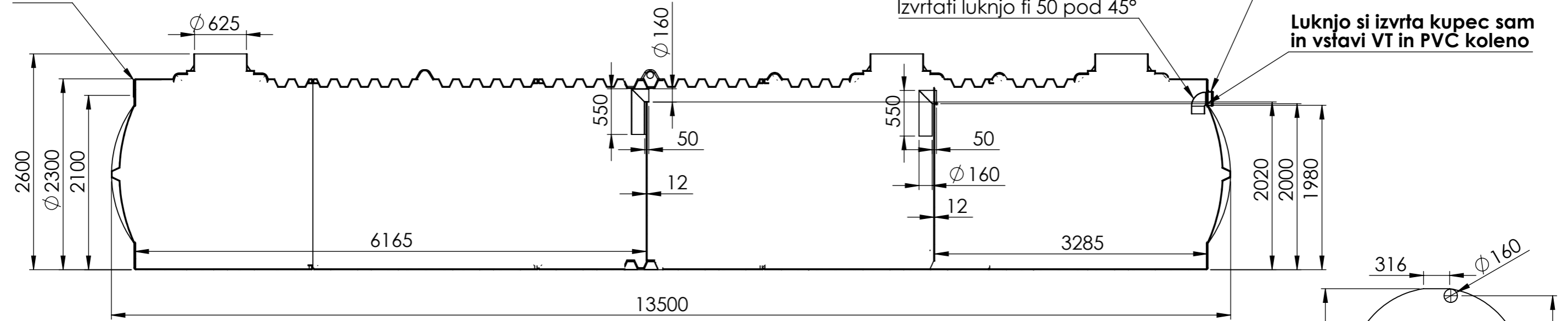
SECTION B-B SCALE 1 : 50
