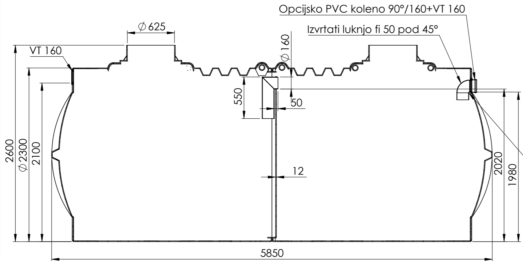
SECTION A-A
